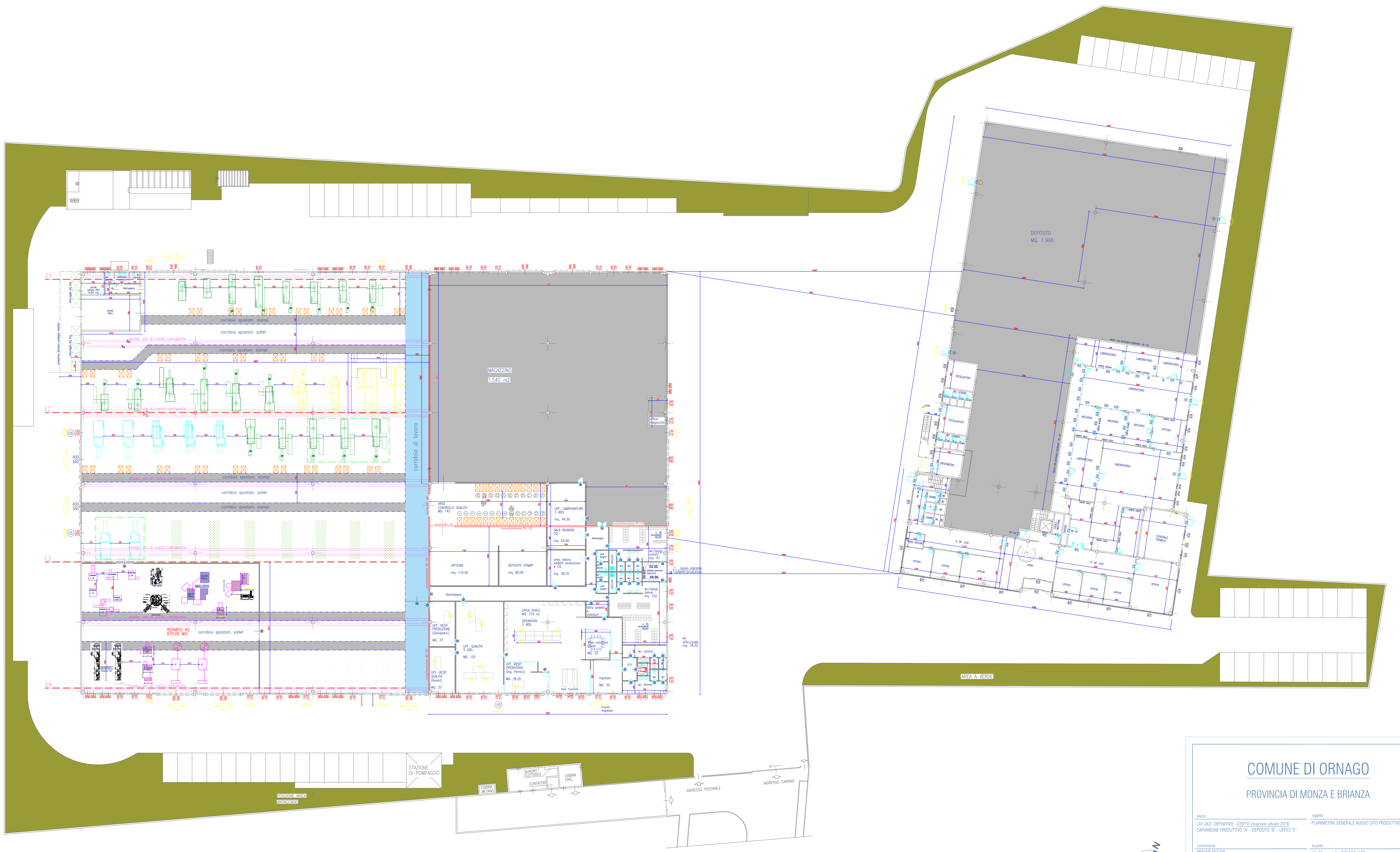
PLANIMETRIA CAPANNONE "A" - PIANO TERRA
