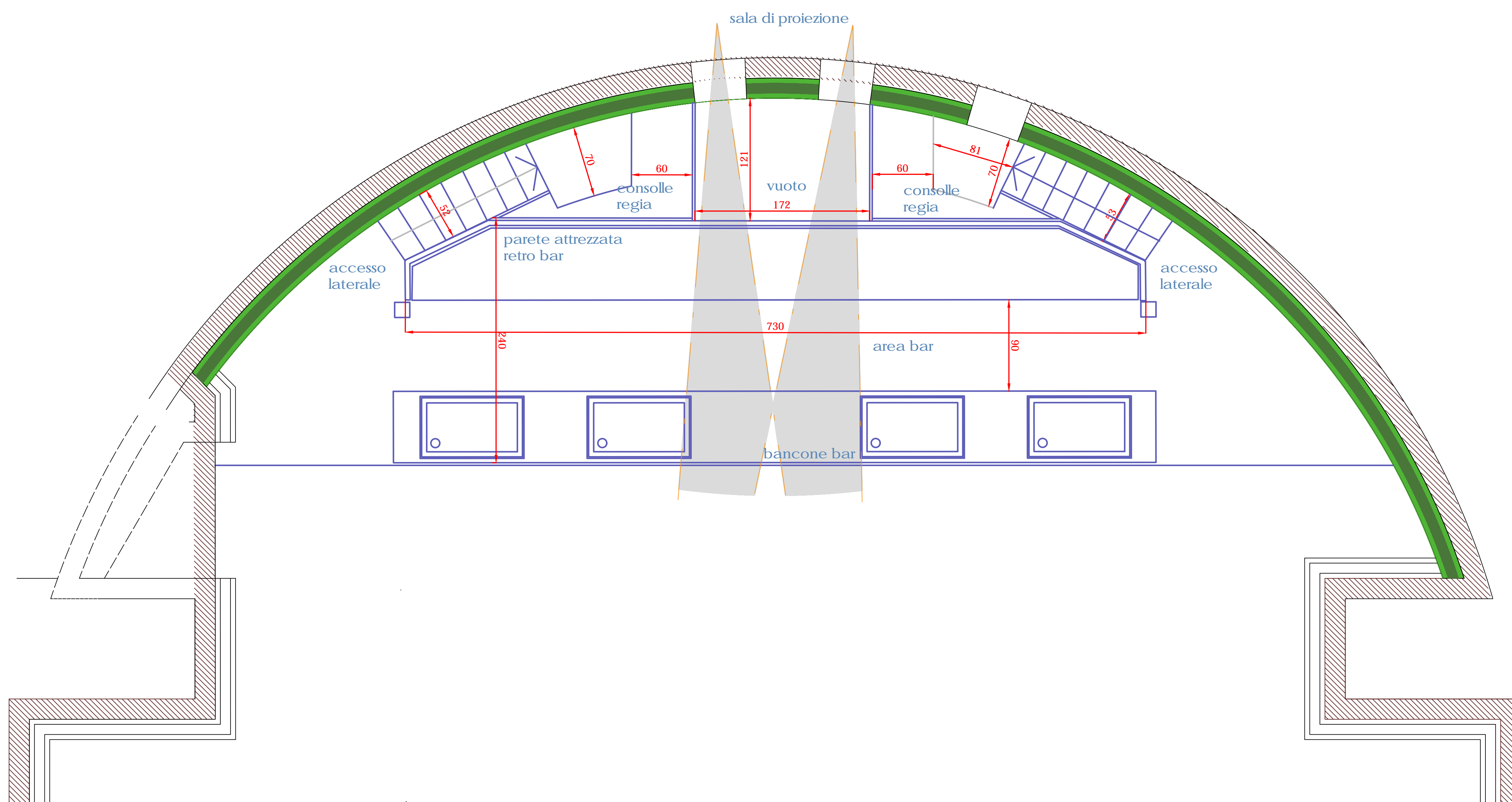
PARTICOLARE PLANIMETRIA ZONA BAR - proposta nuova postazione consolle regia scala 1:25
