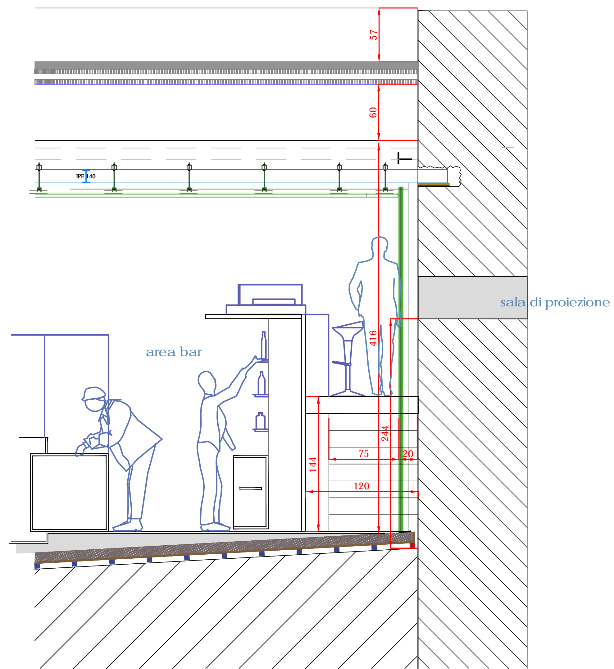
PARTICOLARE SEZIONE RETRO BAR - proposta postazione consolle regia scala 1:25
